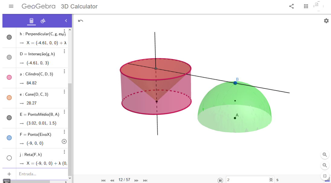
Figura 4.21: Construção da semianticlépsidra
