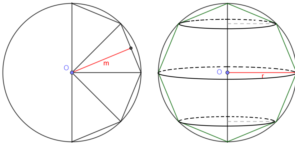
Figura 3.8: Rotação de um polígono regular inscrito em uma circunferência
