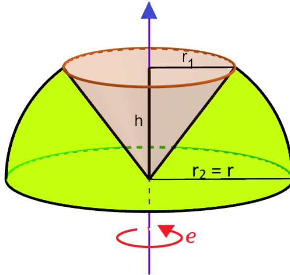
Figura 2.29: Setor esférico do 1º caso
