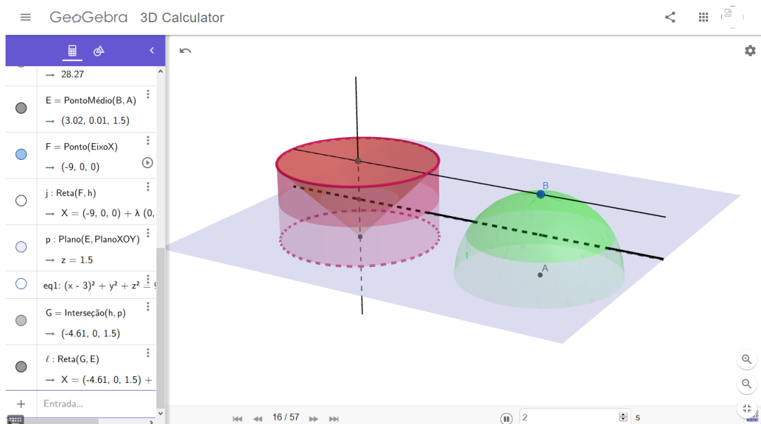
Figura 4.22: Determinação do plano secante à semiesfera e à semianticlépsidra
