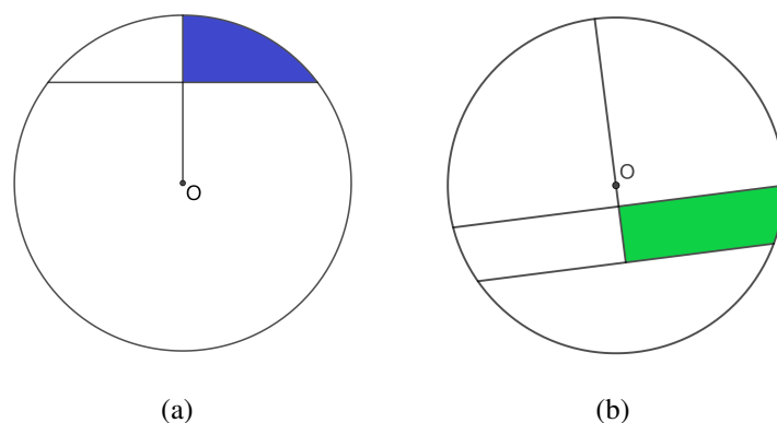
Figura 2.22: Semisegmento circular: (a) de uma base; (b) de duas bases
