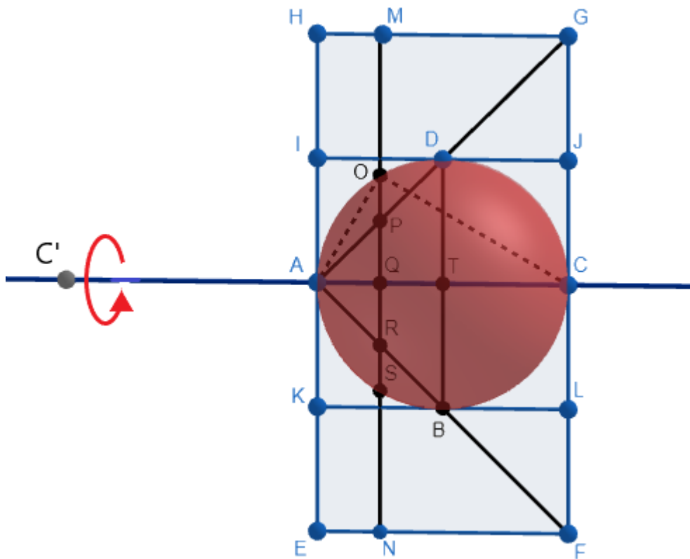
Figura 2.13: Rotação do quadrado ACGH em torno do eixo CC'
