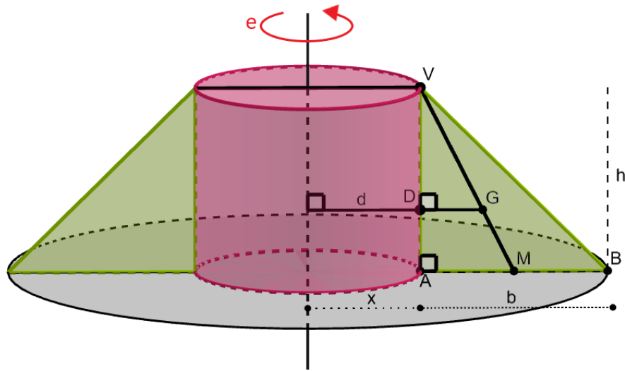
Figura 2.8: Rotação de um triângulo retângulo em torno do eixo e
