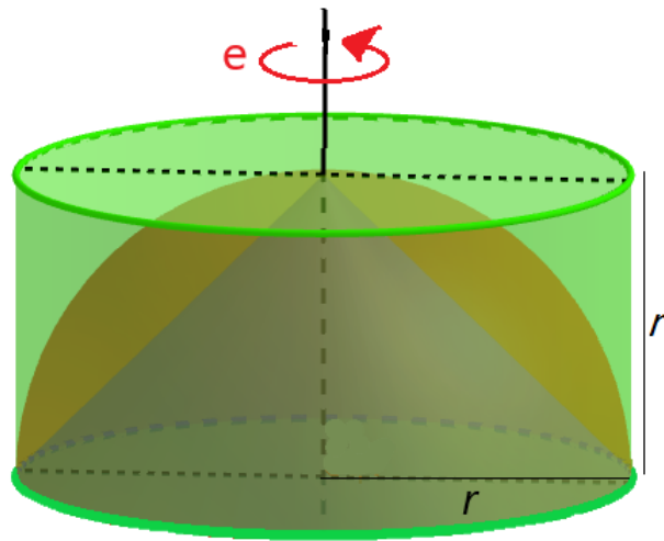
Figura 2.10: Relação entre os volumes do cilindro, da esfera e do cone
