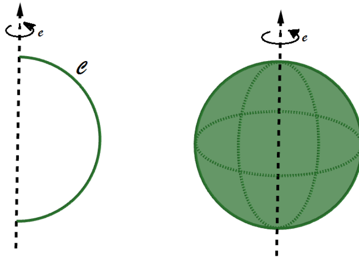
Figura 3.1: A superfície esférica como superfície de revolução
