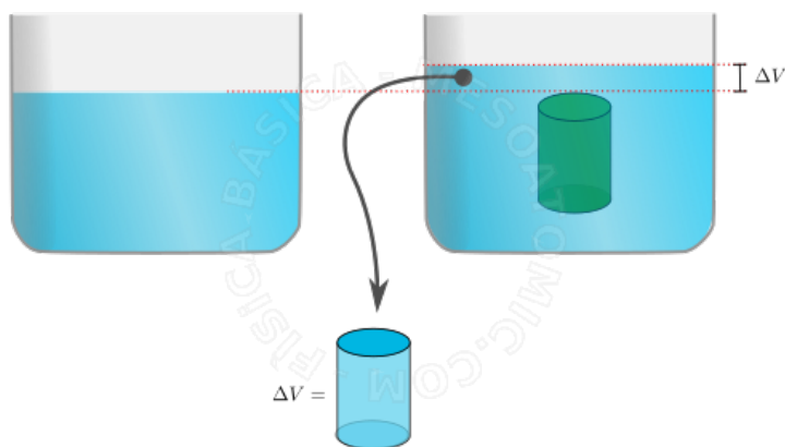
Figura 4.12: Volume de um sólido por imersão
