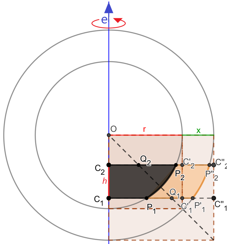
Figura 3.12: Seção em duas esferas concêntricas
