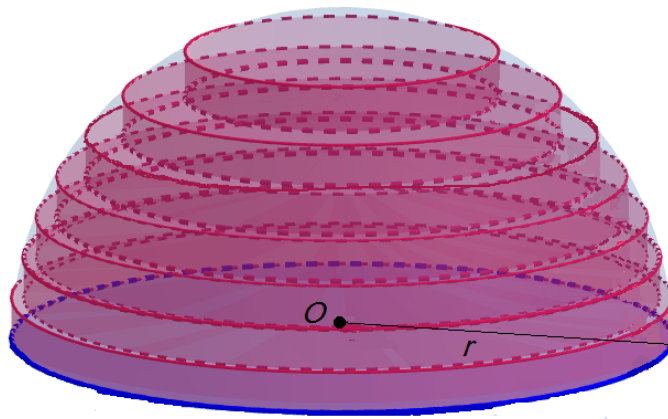
Figura 2.16: Semiesfera com cilindros retos inscritos
