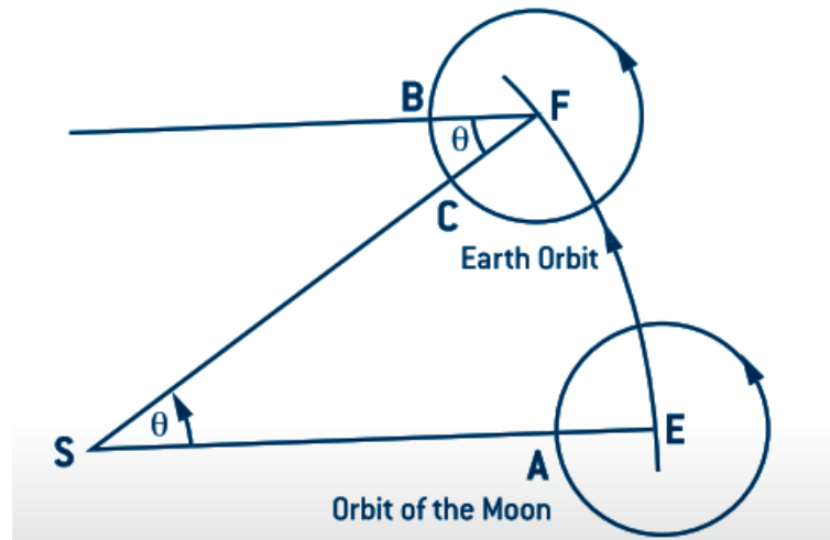
Figura 4.8: Relação entre o Sol, a Lua e a Terra de um ponto de vista geométrico
