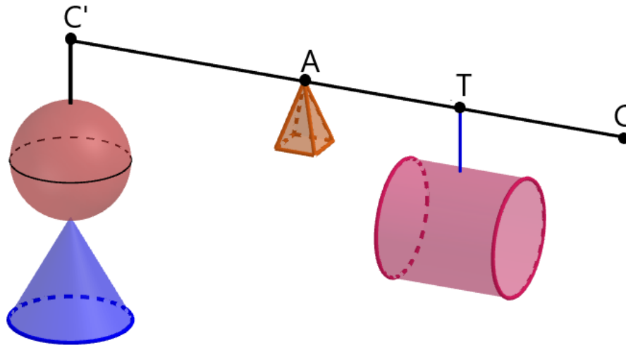
Figura 2.14: Relação entre o volume do cone, da esfera e do cilindro pelo princípio de equilíbrio de Arquimedes
