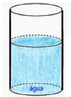
Figura 4.15: Recipiente cilíndrico com água para imersão dos sólidos
