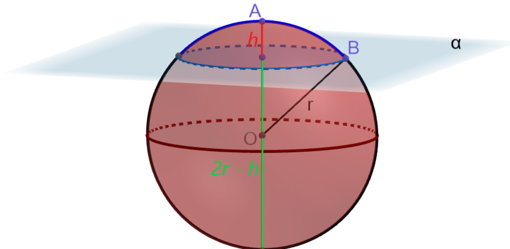
Figura 3.13: Calotas esféricas de alturas h e 2r - h
