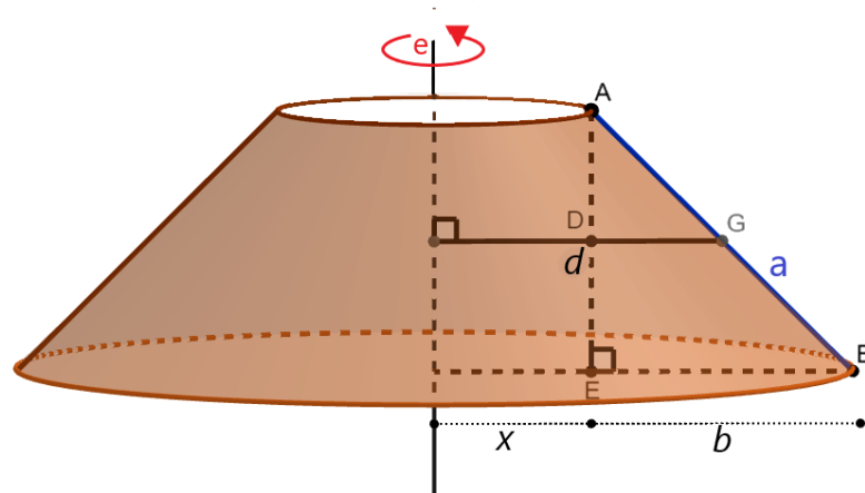
Figura 3.6: Rotação de um segmento de reta \overline{AB} em torno do eixo e
