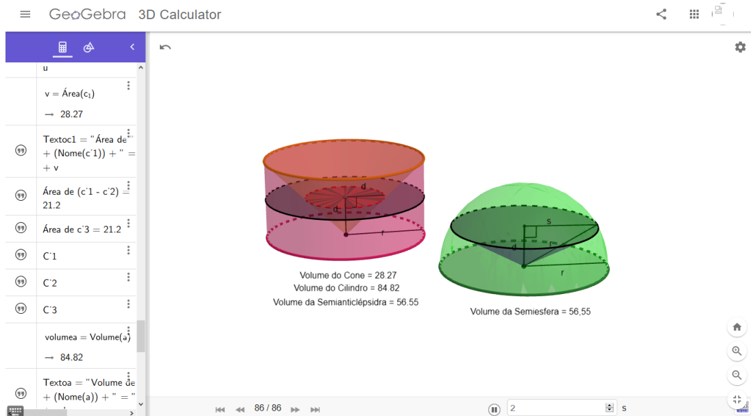
Figura 4.25: Volume da semiesfera e da semianticlépsidra
