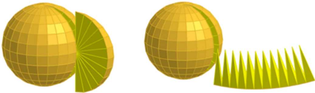
Figura 3.4: Esfera decomposta em pirâmides
