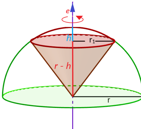
Figura 2.31: Setor esférico do 3º caso
