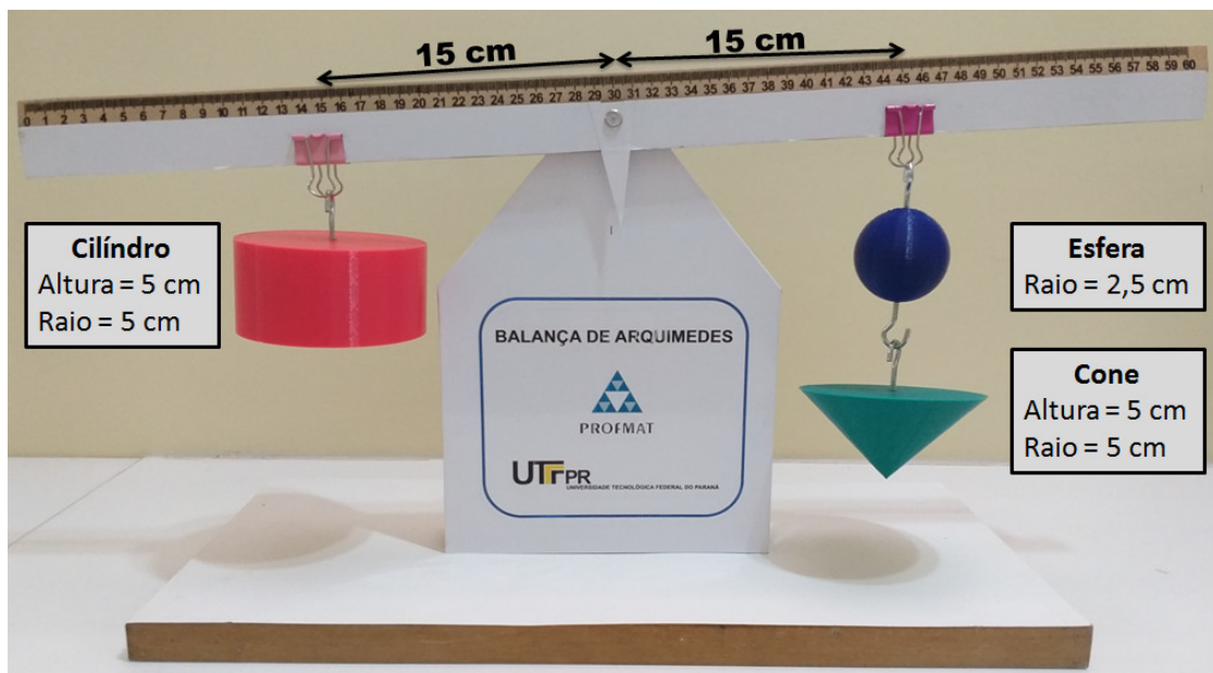
Figura 4.18: Balança de Arquimedes em desequilíbrio
