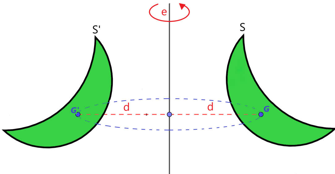
Figura 2.7: Rotação da figura S em torno do eixo e
