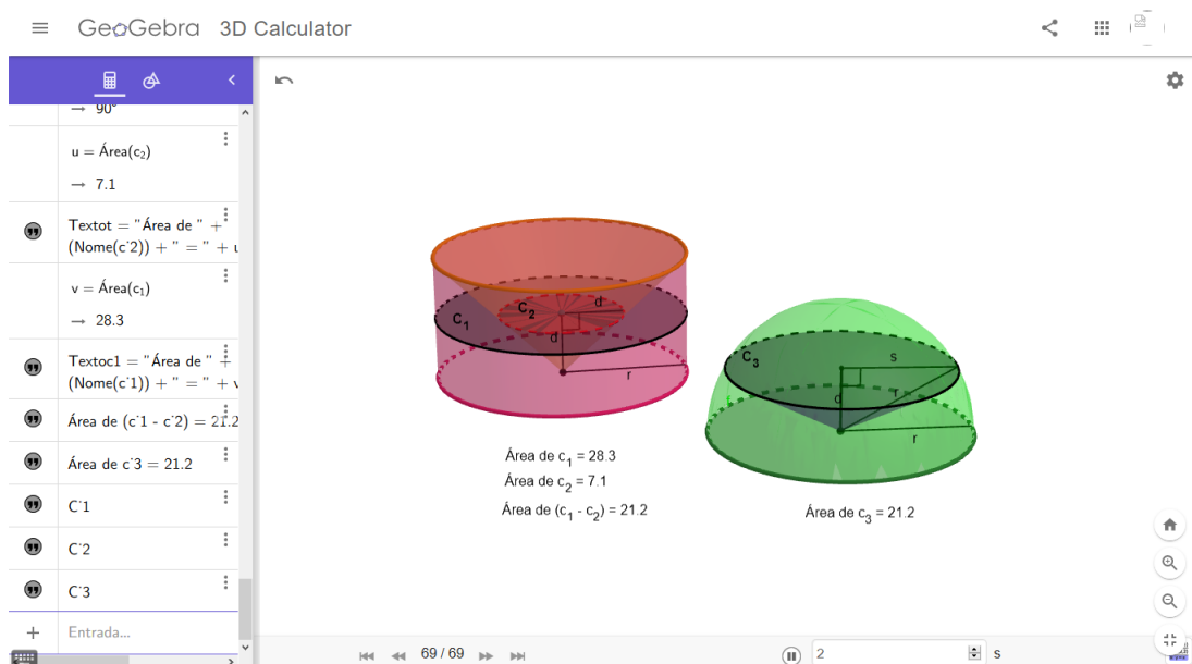
Figura 4.24: Área das seções na semiesfera e na semianticlépsidra
