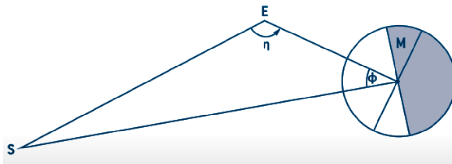
Figura 4.10: O elongamento da Lua
