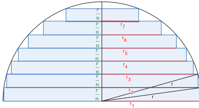
Figura 2.17: Raios dos cilindros retos inscritos na semiesfera
