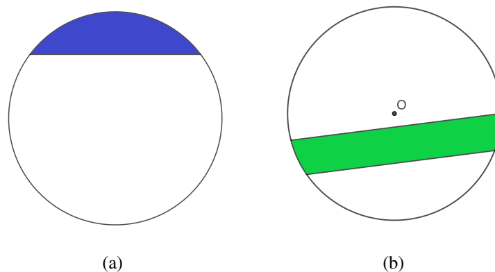
Figura 2.21: Segmento circular: (a) de uma base; (b) de duas bases
