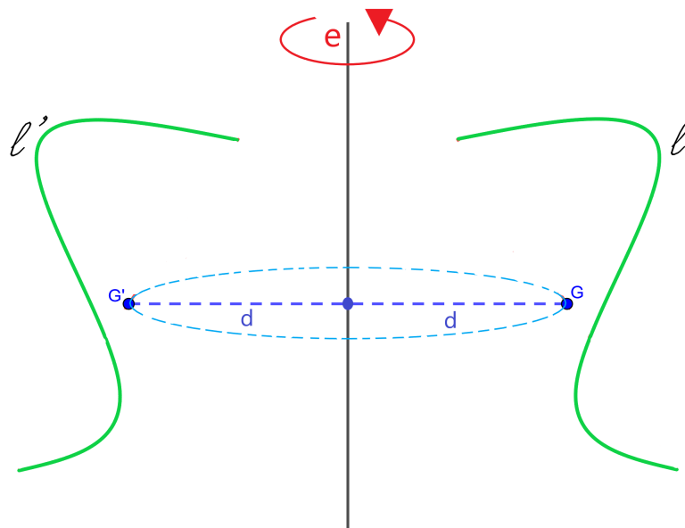
Figura 3.5: Rotação da linha \ell em torno do eixo e
