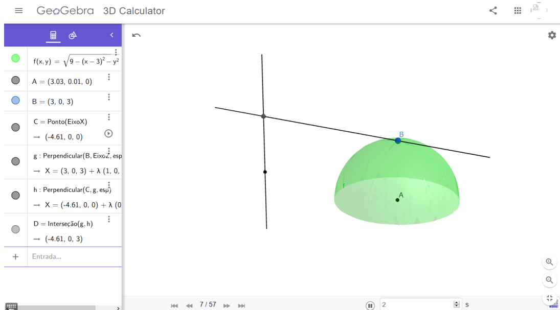
Figura 4.19: Construção da semiesfera de raio \overline{AB} = 3\text{ cm}
