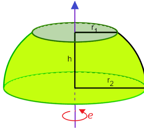
Figura 2.24: Segmento esférico de duas bases de raios r_1 e r_2 e altura h
