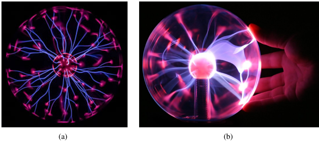
Figura 4.4: Globo de plasma: (a) em funcionamento; (b) reação ao toque de uma pessoa
