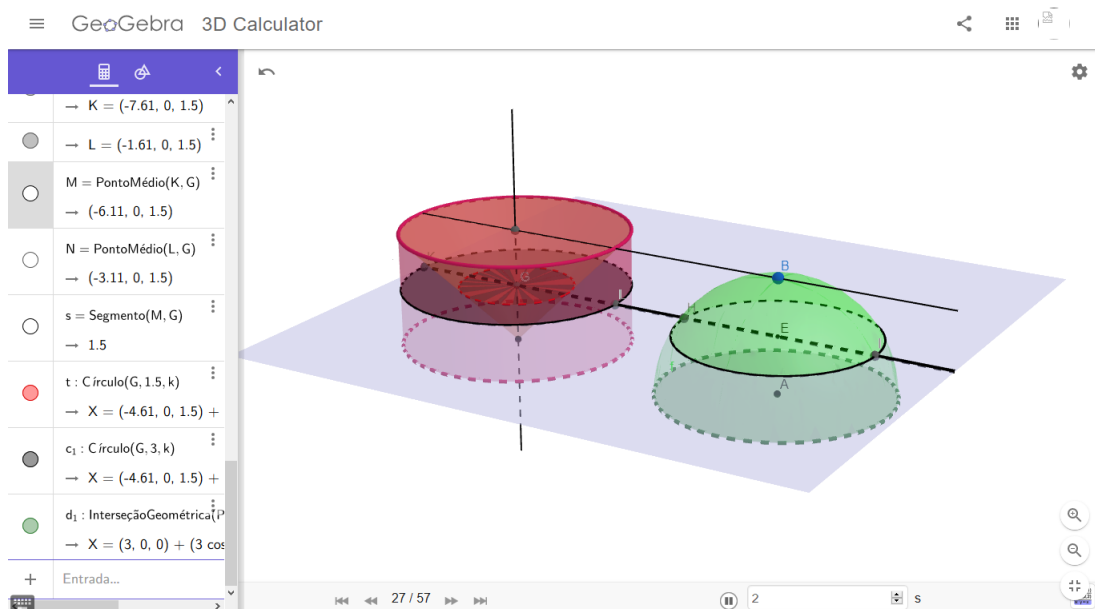
Figura 4.23: Seções na semiesfera e na semianticlépsidra
