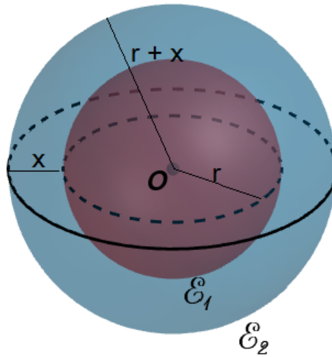
Figura 3.3: Esferas concêntricas \mathcal{E}_1 e \mathcal{E}_2 de raios respectivamente iguais a r e r+x
