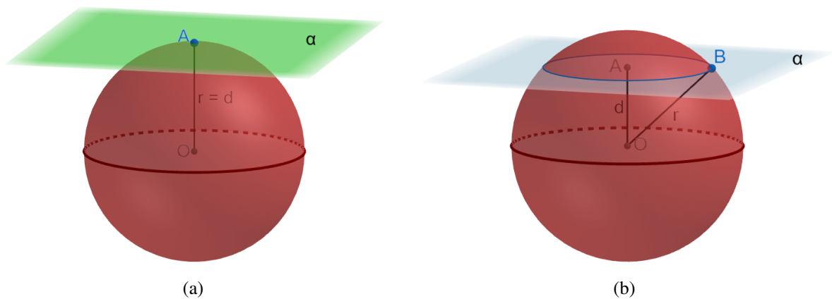
Figura 2.20: Plano \alpha : (a) tangente à esfera de centro O e raio r ; (b) secante à esfera de centro O e raio r
