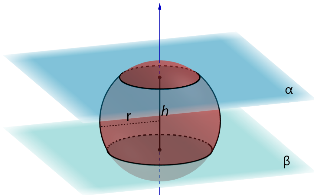
Figura 3.11: Zona esférica de altura h
