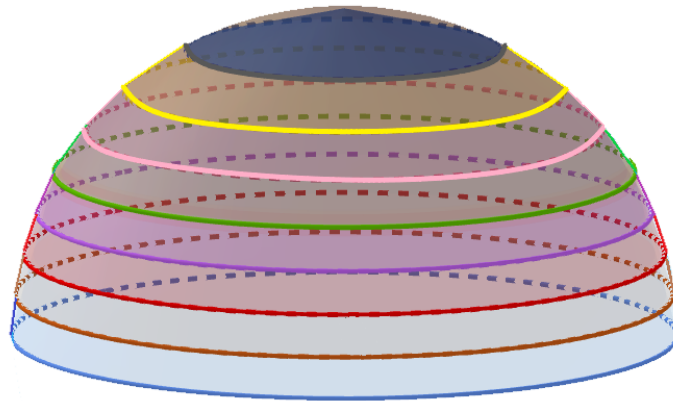
Figura 2.18: Semiesfera com troncos de cone retos de bases paralelas inscritos
