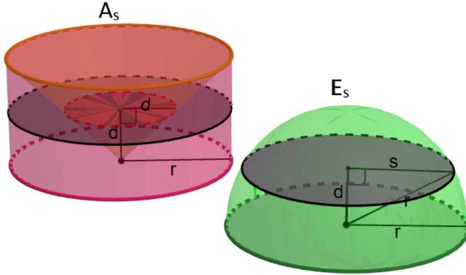
Figura 2.5: Semianticlépsidra e semiesfera equivalentes
