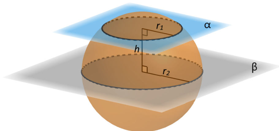
Figura 2.25: Segmentos esféricos determinados por dois planos paralelos \alpha e \beta secantes à esfera
