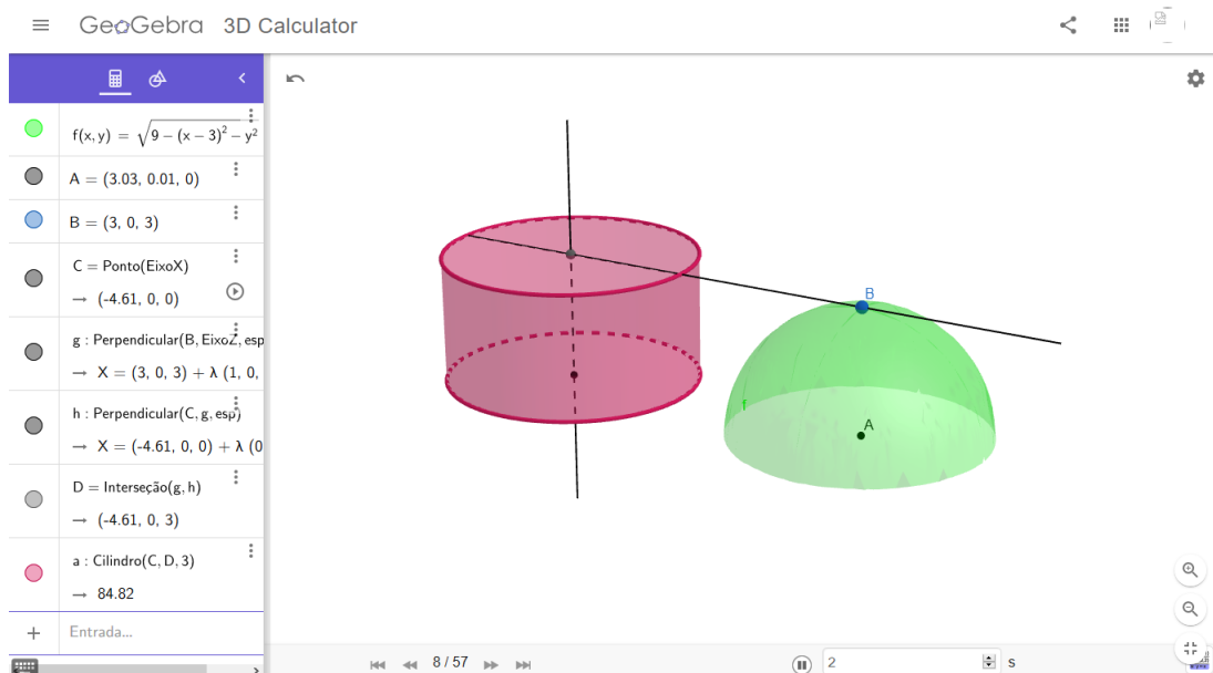
Figura 4.20: Construção do cilindro de altura \overline{AB} = 3\text{ cm} e raio r = 3\text{ cm}
