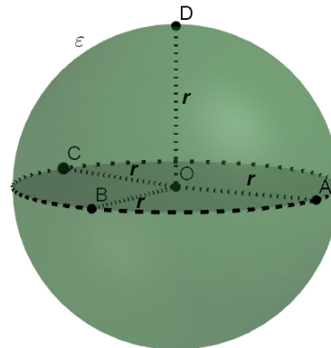
Figura 2.1: Esfera de centro O e raio r
