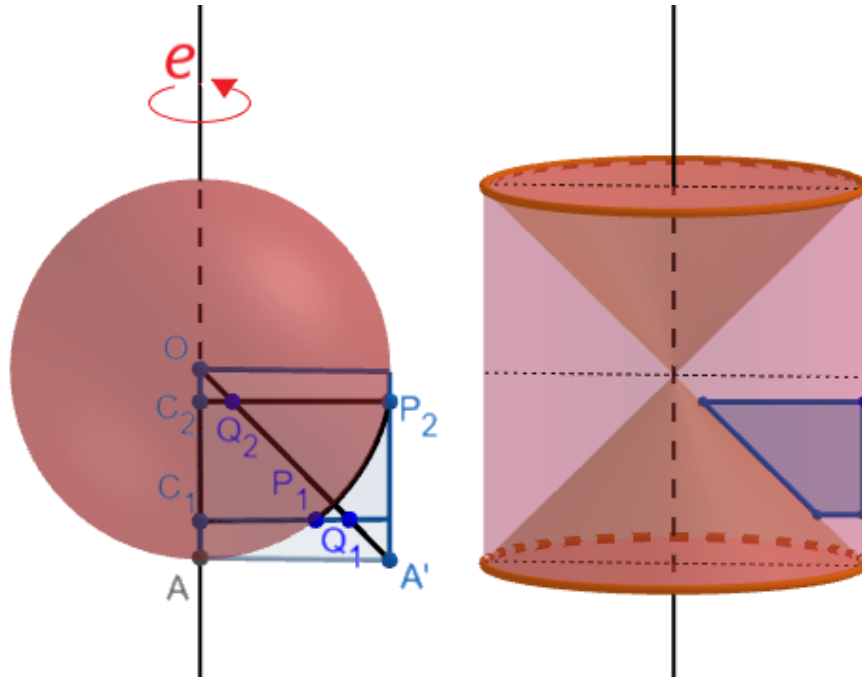
Figura 2.26: Volume do segmento esférico de duas bases na esfera e na anticlépsidra
