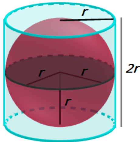
Figura 2.11: Esfera inscrita em um cilindro equilátero
