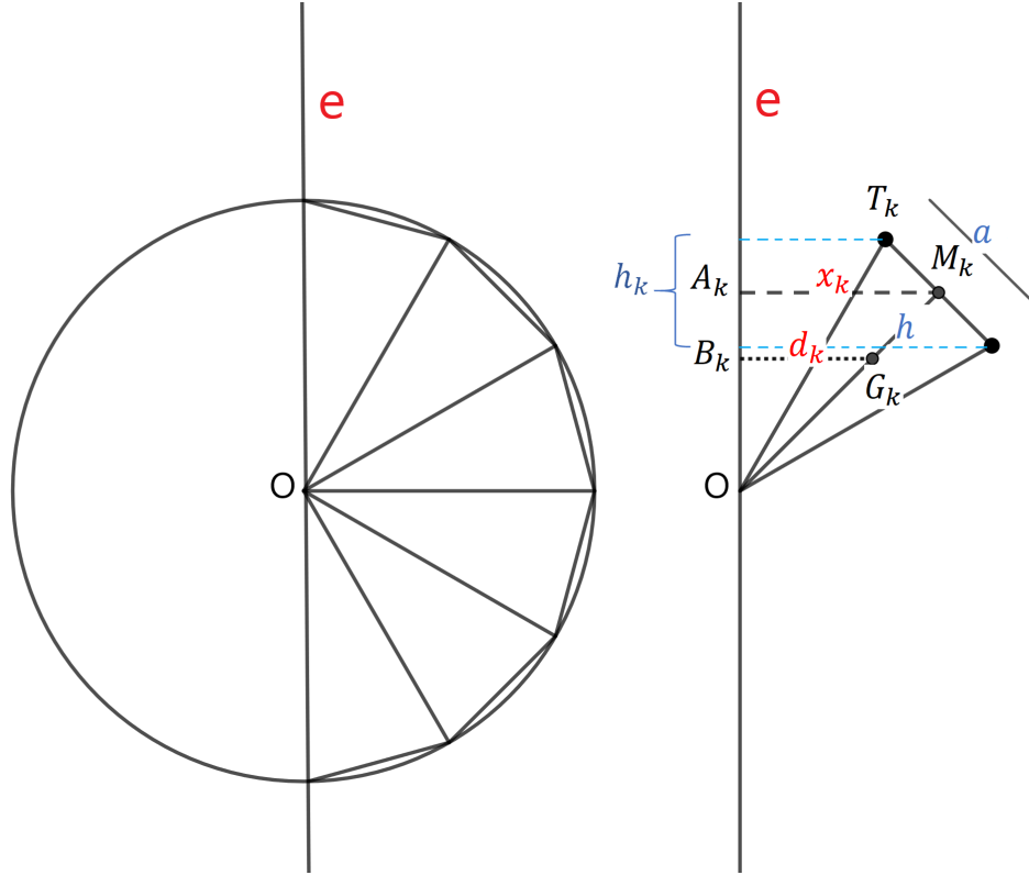
Figura 2.9: Rotação de um semicírculo em torno do eixo e para gerar a esfera
