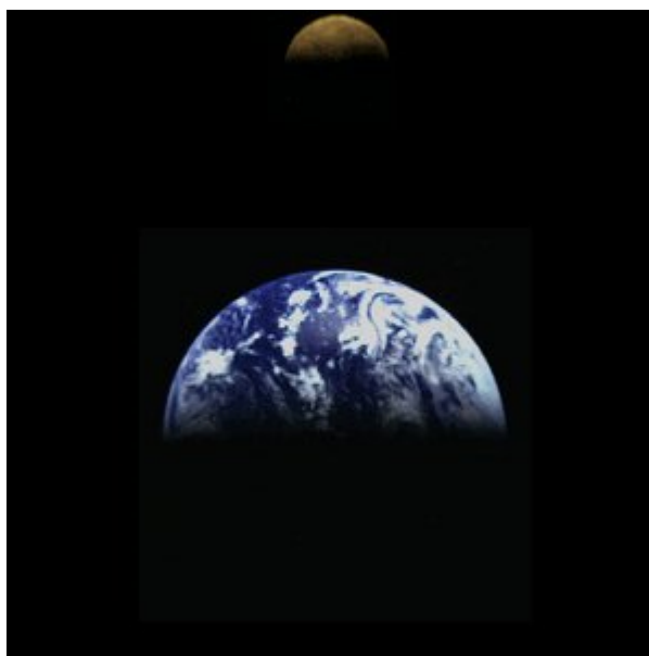
Figura 4.6: Face da Lua iluminada pelo Sol
