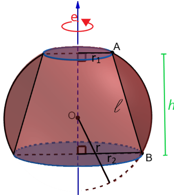
Figura 2.34: Anel esférico do 2º caso
