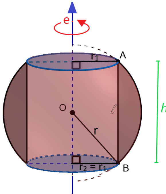
Figura 2.33: Anel esférico do 1º caso
