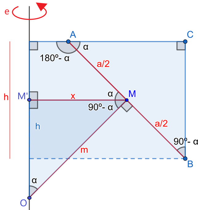
Figura 2.6: Segmento \overline{AB} disjunto do eixo e
