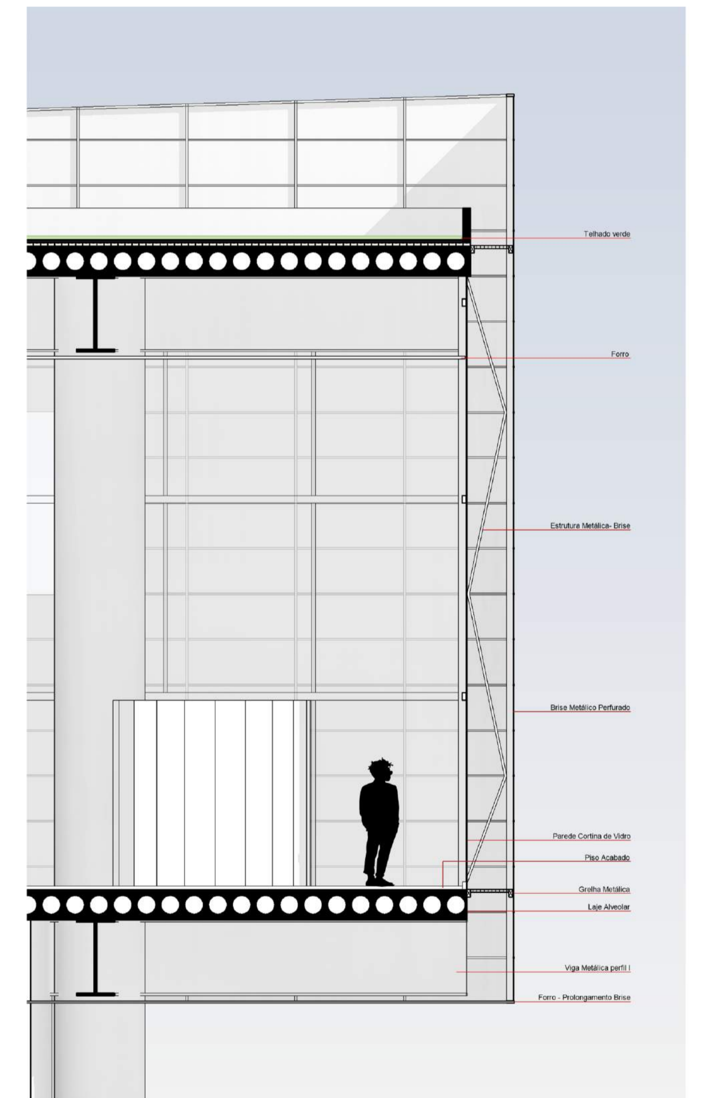
DETALHE 01 ESCALA 1:50
