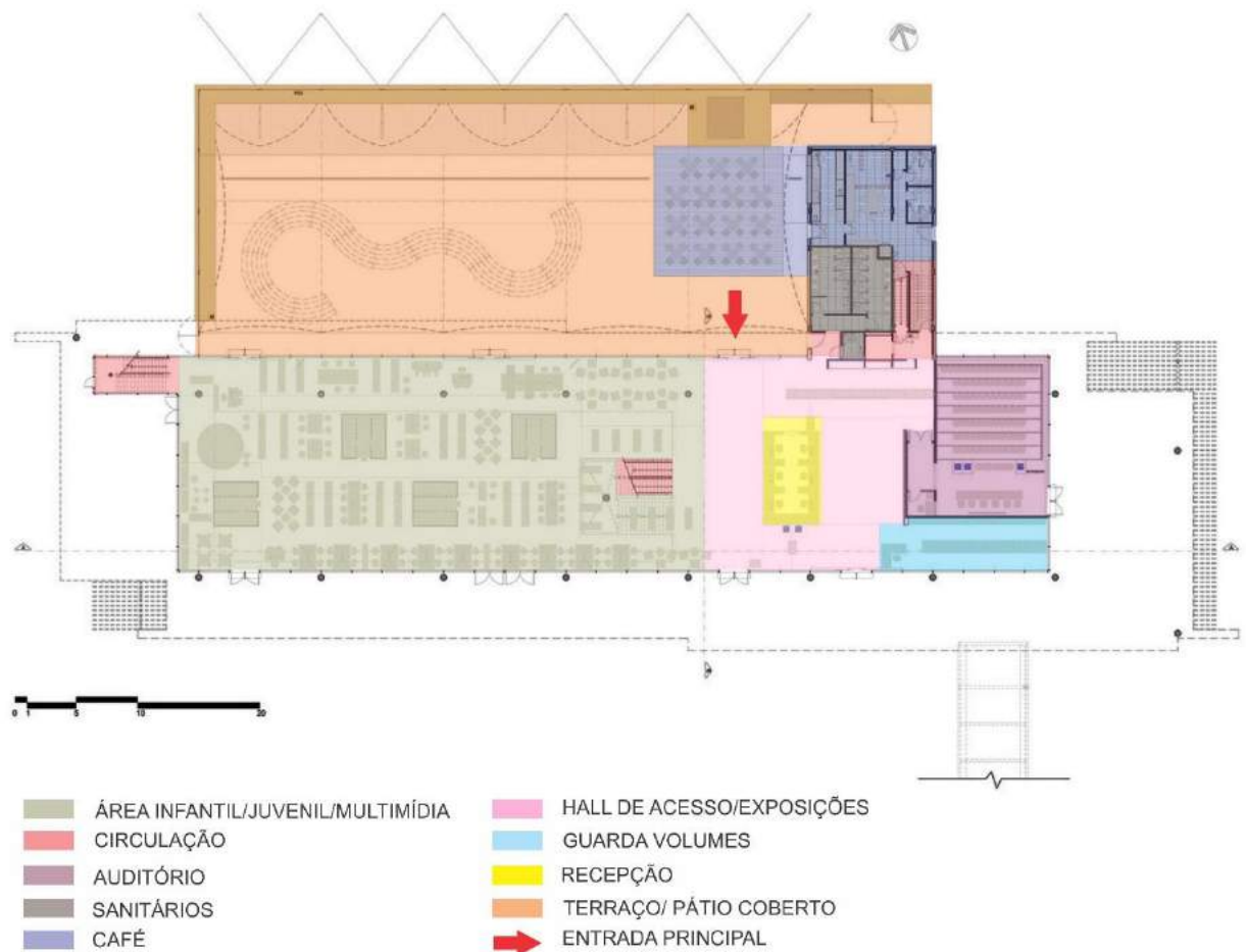
Figura 16- Biblioteca São Paulo – planta do pavimento térreo. Fonte: archdaily.com.br
