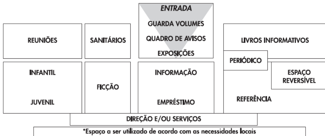
Figura 5- Relação das áreas de uma biblioteca: sugestão de fluxo. Fonte: Fundação Biblioteca Nacional, 2010.
