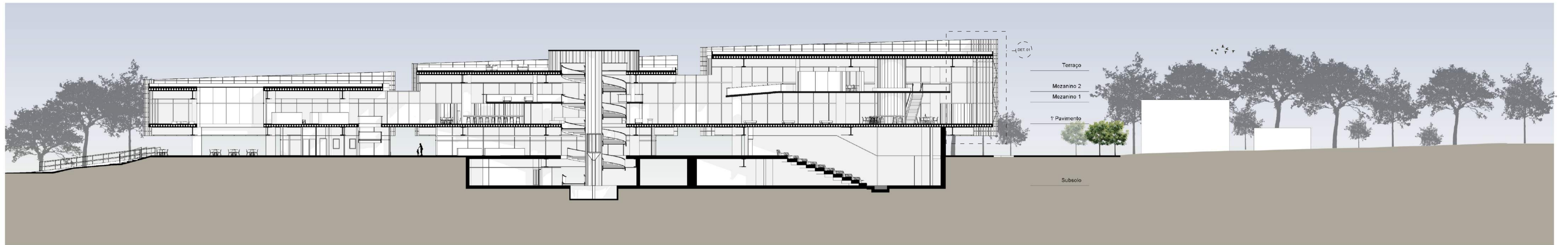
CORTE A ESCALA 1:250
