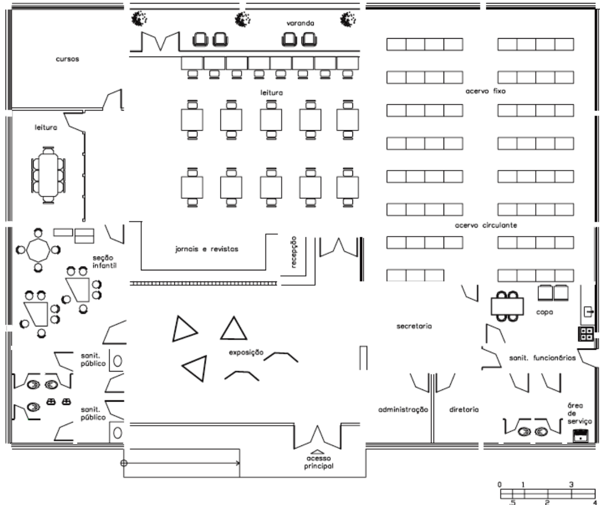
Figura 6 - Exemplo de planta. Fonte Fundação Biblioteca Nacional, 2010.
