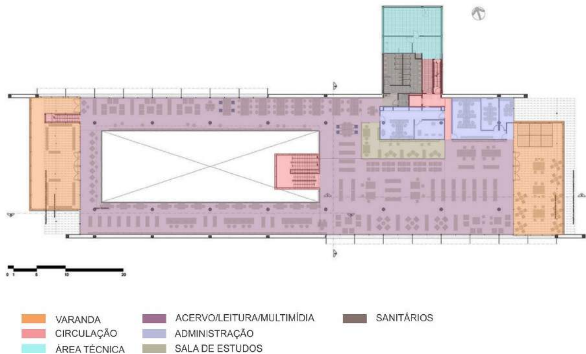
Figura 17- Biblioteca São Paulo – planta do segundo pavimento. Fonte: archdaily.com.br
